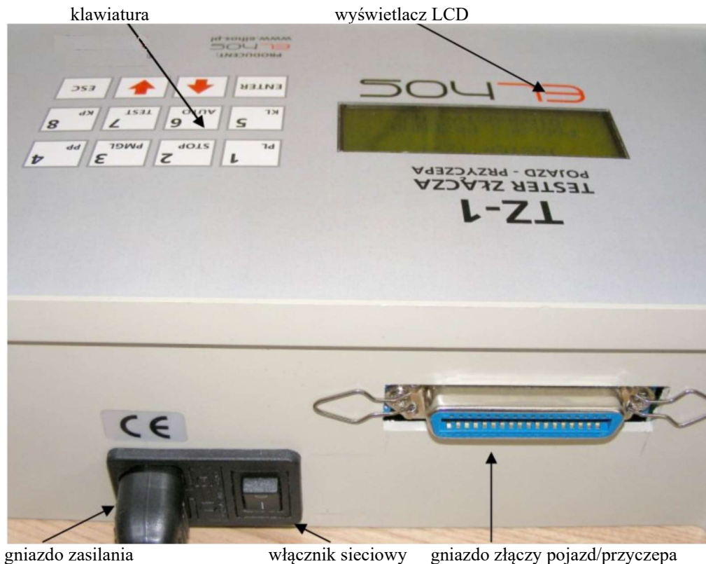
Rys 3. Przykładowe urządzenie
